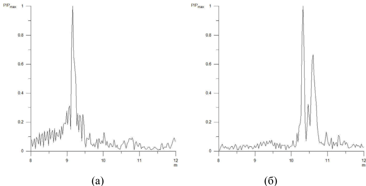
Рис.4. – Примеры экспериментальных распределений модуля мощности эхосигналов по дальности, при корреляционной обработке ЛЧМ сигналов акустического маяка
